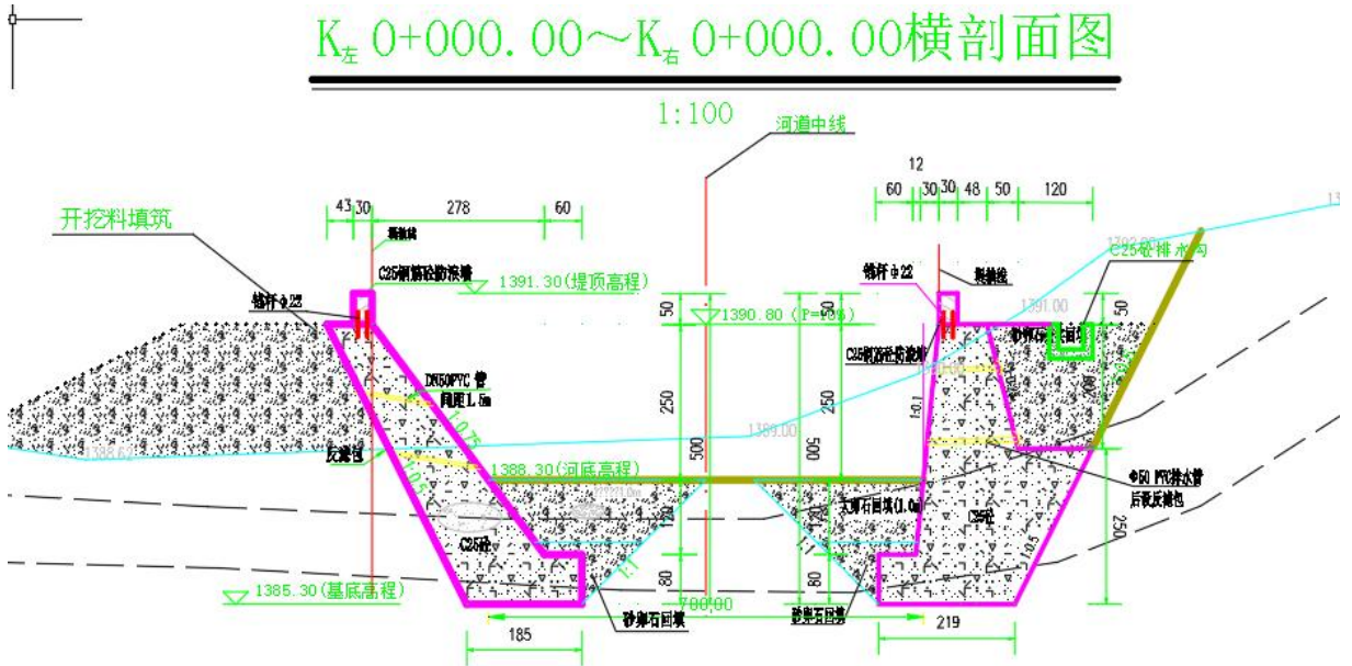
图 2-3 本项目河堤 1 典型断面堤防剖面图
