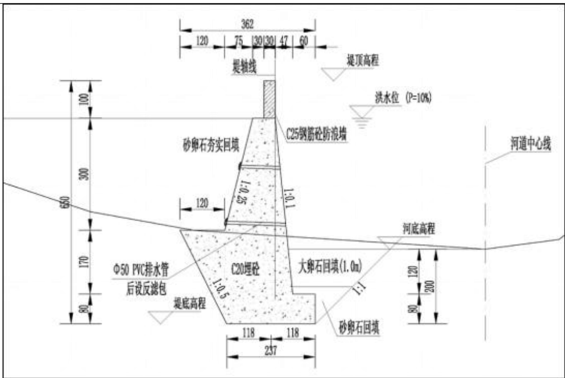
图 2-2 衡重式堤防典型面图
