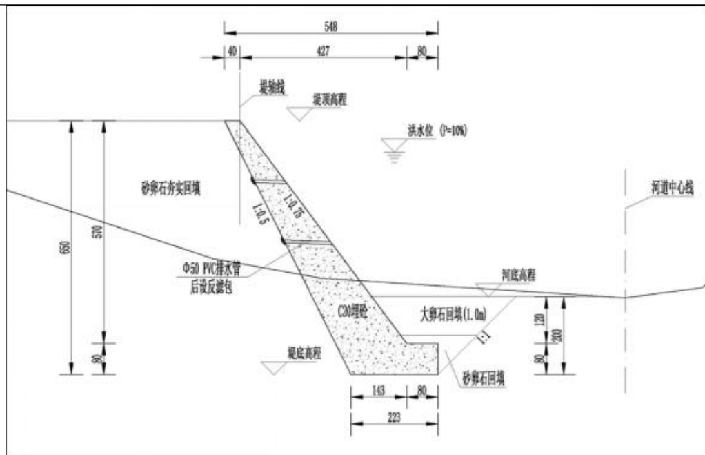
图 2-1 仰斜式堤防典型面图
