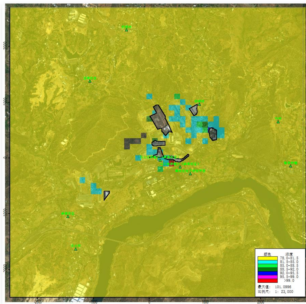
图 2-10 叠加后 PM 10 保证率日平均网格浓度分布图 单位: \mu\text{g}/\text{m}^3
