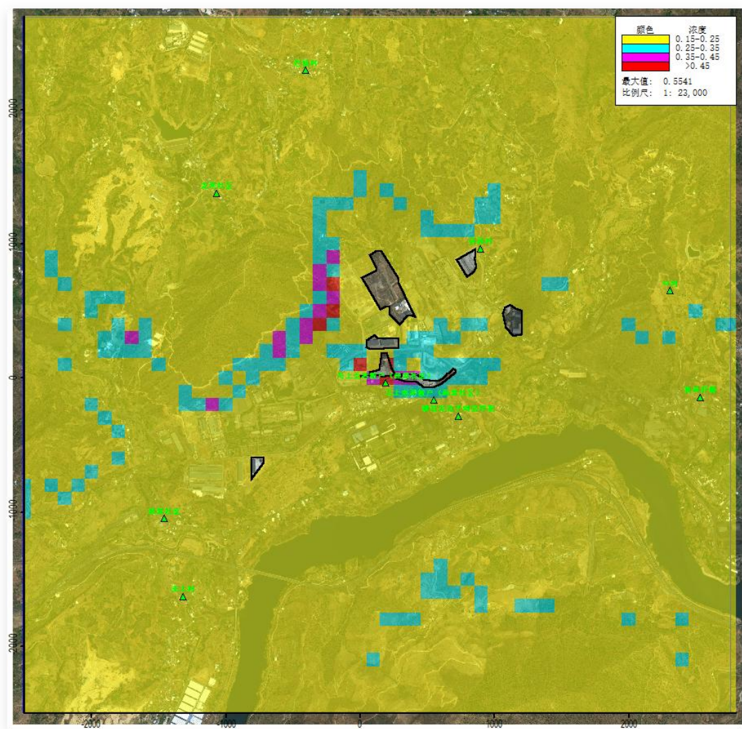
图 2-19 叠加后氟化物日平均网格浓度分布图 单位：μg/m 3
