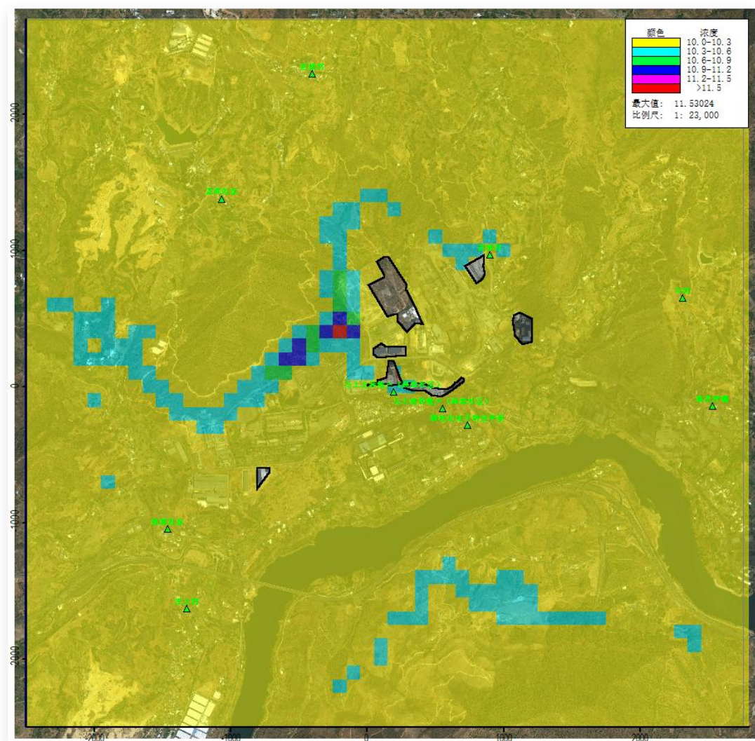
图 2-21 叠加后 HCl 日平均网格浓度分布图 单位：μg/m³
