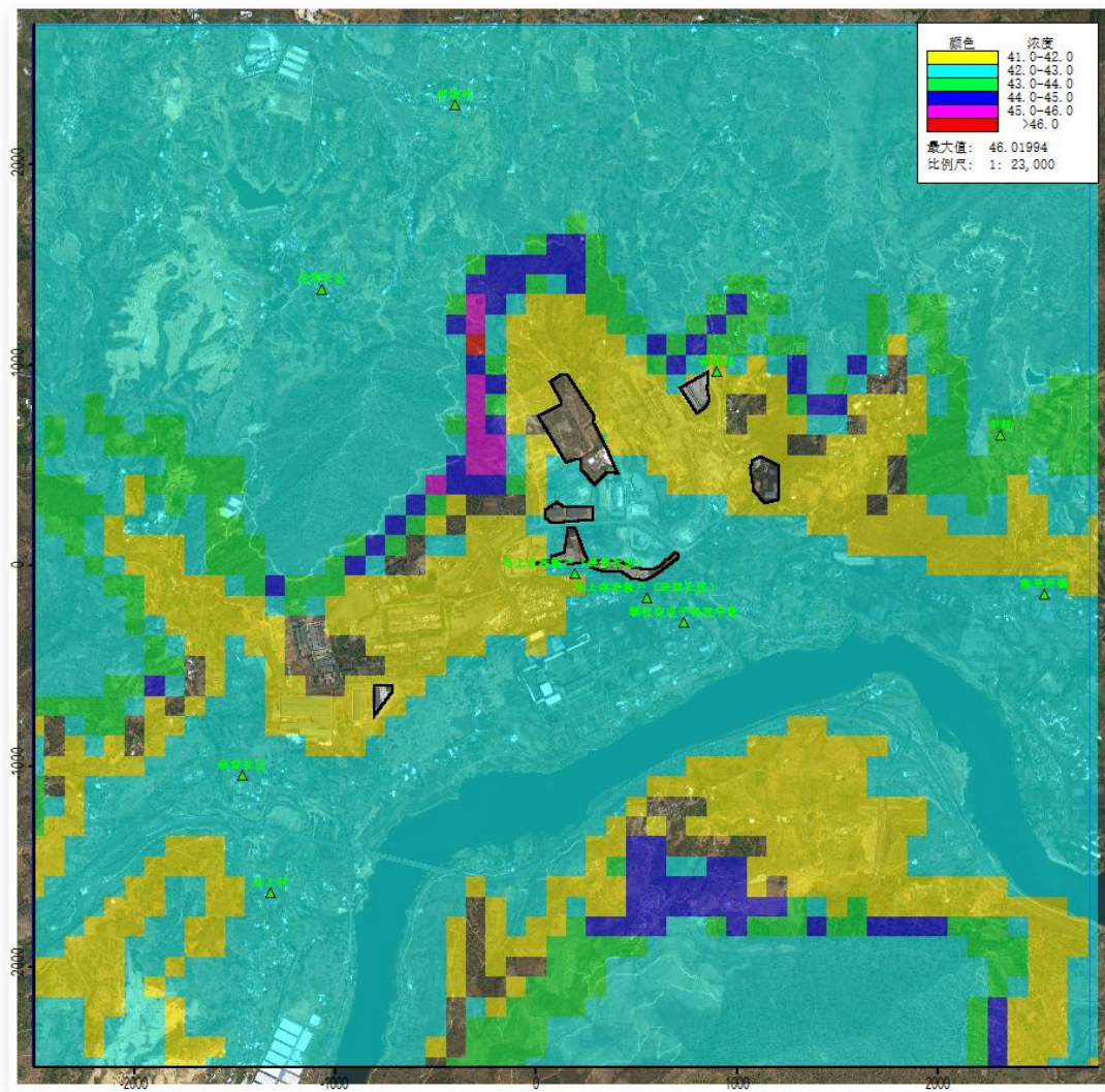
图 2-16 叠加后 NO 2 保证率日平均网格浓度分布图 单位: \mu\text{g}/\text{m}^3
