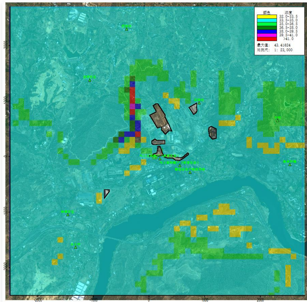
图 2-14 叠加后 SO 2 保证率日平均网格浓度分布图 单位： \mu\text{g}/\text{m}^3
