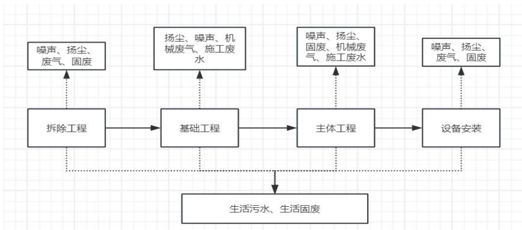
图 2-3 施工期工艺流程及产排污分布图
