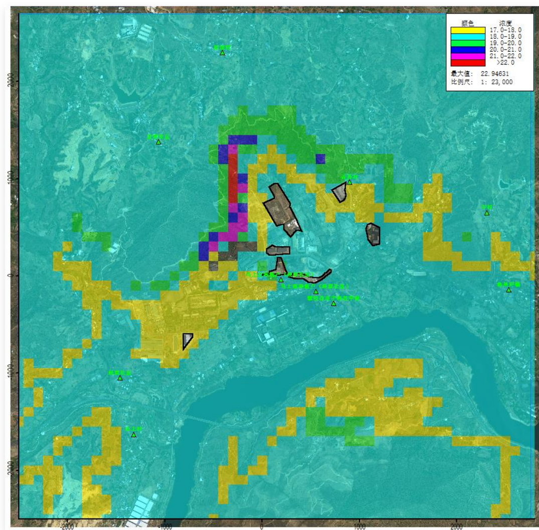
图 2-15 叠加后 SO 2 年平均网格浓度分布图 单位：µg/m 3
