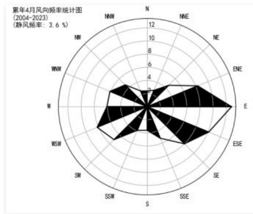
4 月静风 3.6%
