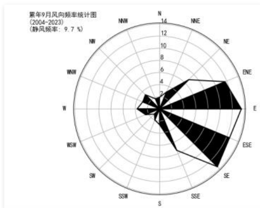
9 月静风 9.7%
