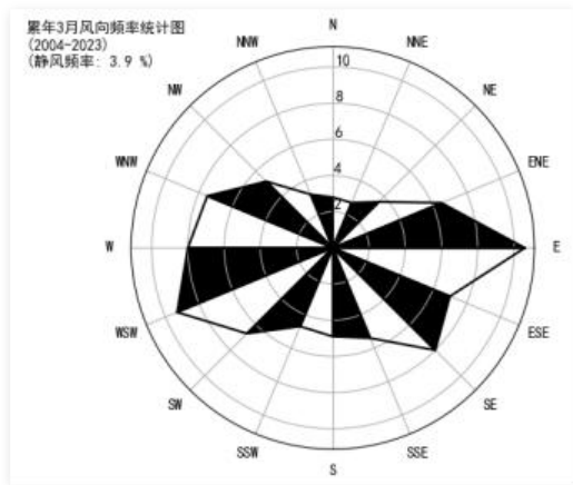
3 月静风 3.9%
