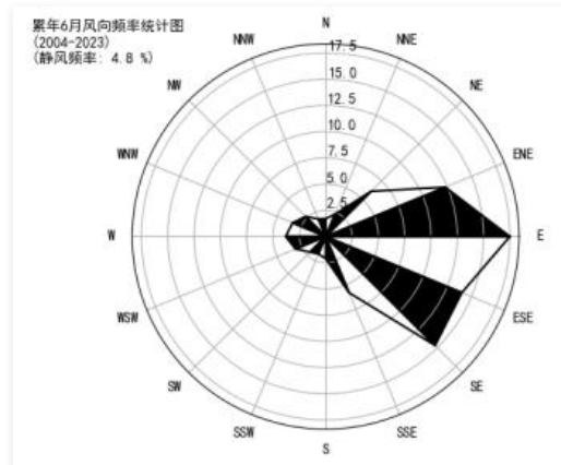
6 月静风 4.8%
