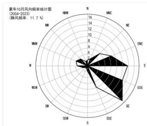
10 月静风 11.7%
