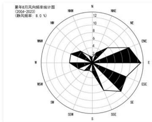
8 月静风 8.0%
