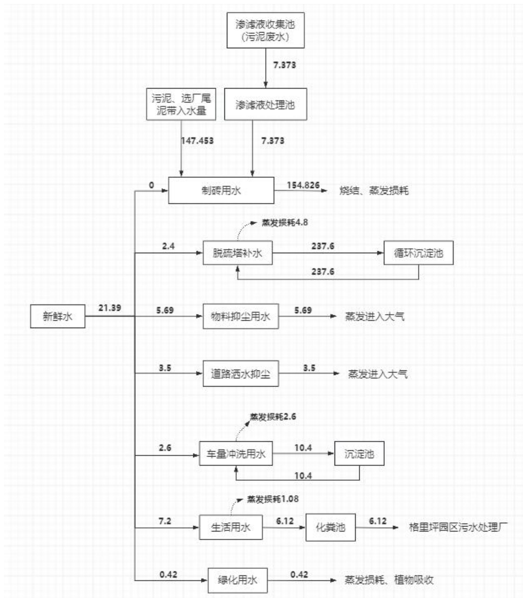
图 2-2 项目全厂水平衡图（单位：m 3 /d）
