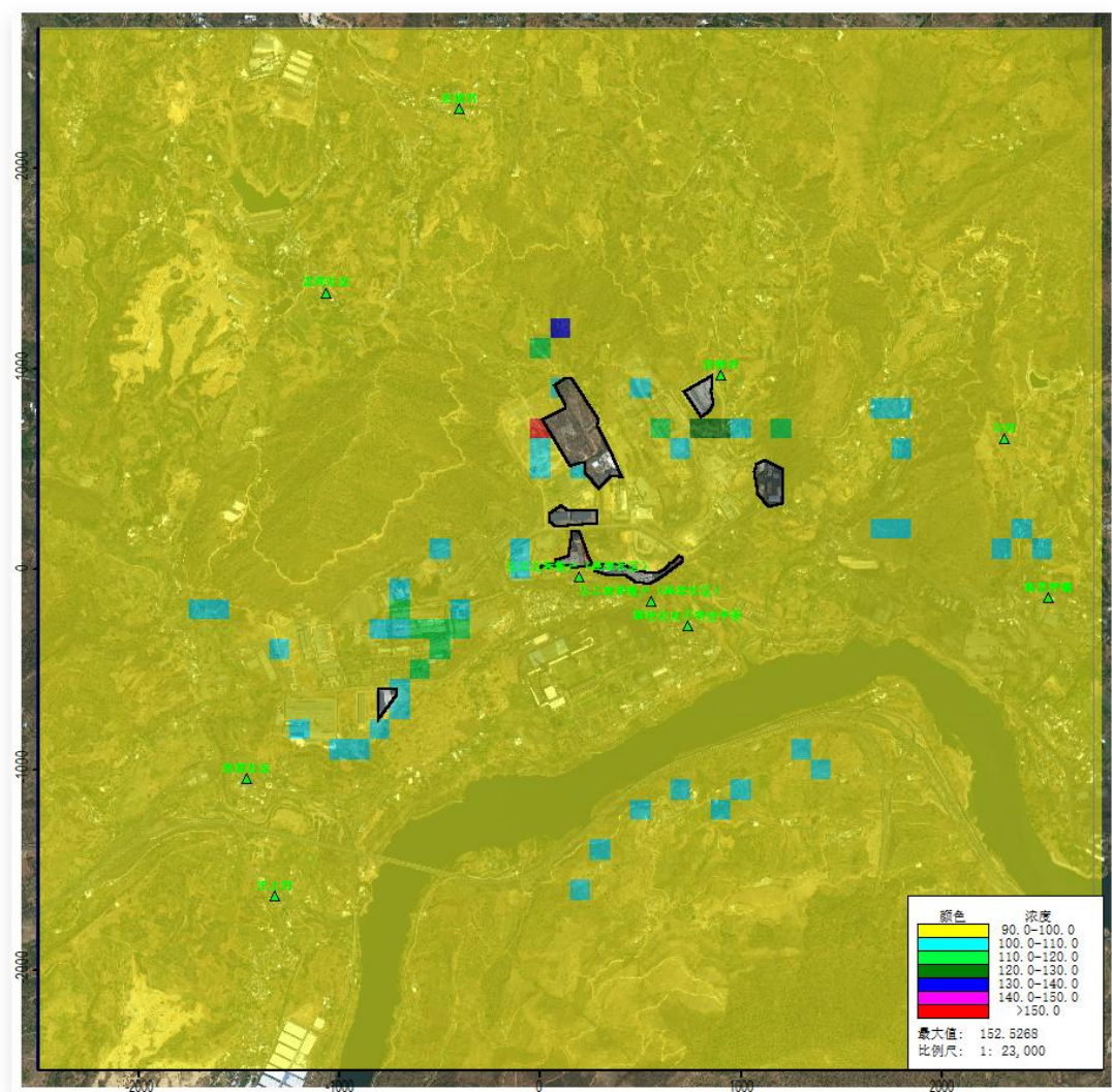
图 2-28 叠加后 NH 3 小时平均网格浓度分布图 单位: \mu\text{g}/\text{m}^3
