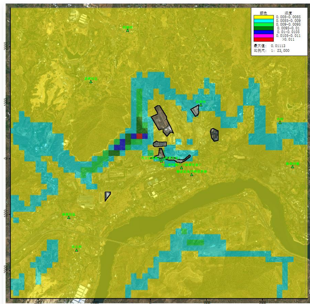
图 2-24 叠加后 As 日平均网格浓度分布图 单位：μg/m³
