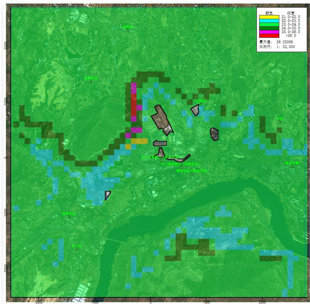
图 2-17 叠加后 NO 2 年平均网格浓度分布图 单位: \mu\text{g}/\text{m}^3
