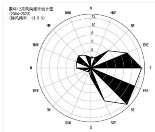
12 月静风 13.5%
