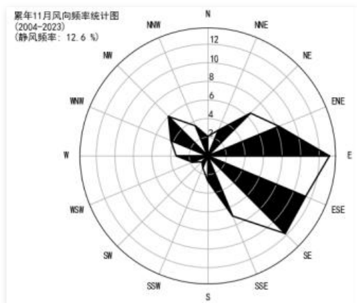
11 月静风 12.6%
