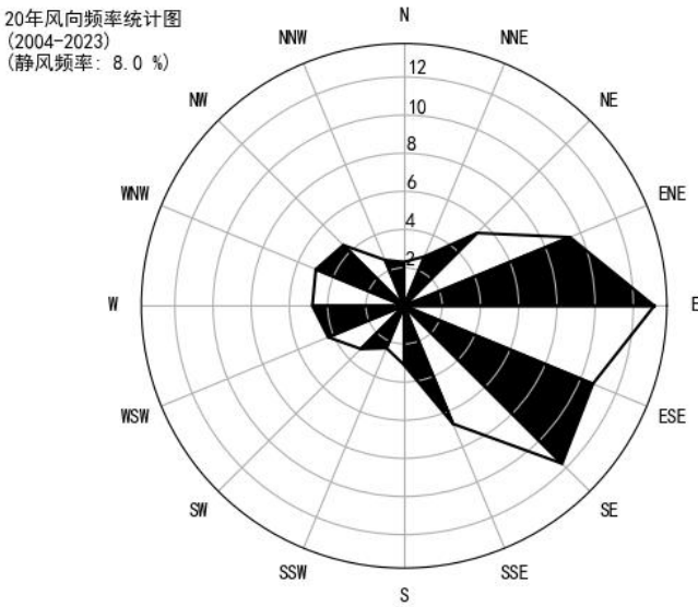
图 2-1 攀枝花气象站风向玫瑰图（静风频率 8.0%）
