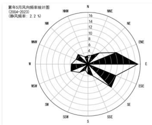
5 月静风 2.2%
