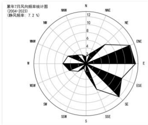
7 月静风 7.2%
