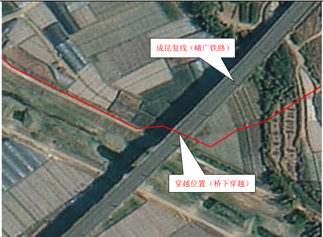
图 2.3.5-1 管道与铁路隧道交叉穿越点平面布置图
