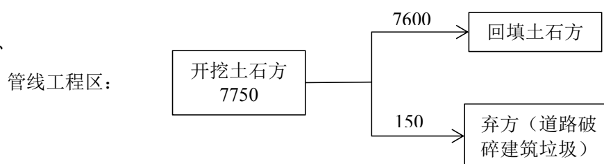
图 2.3.7-1 拟建项目土石方平衡图（单位：m 3 ）
