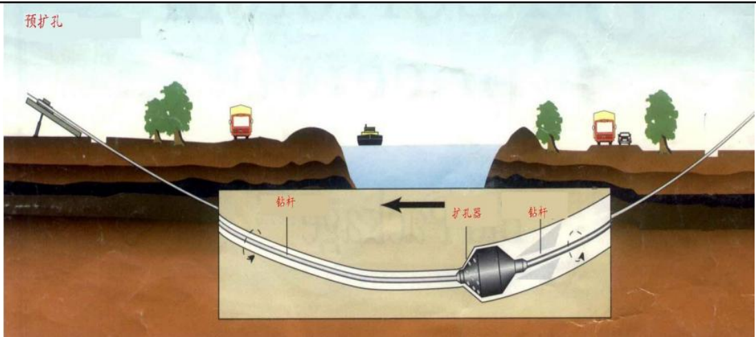
图 2.4-4 扩孔示意图
