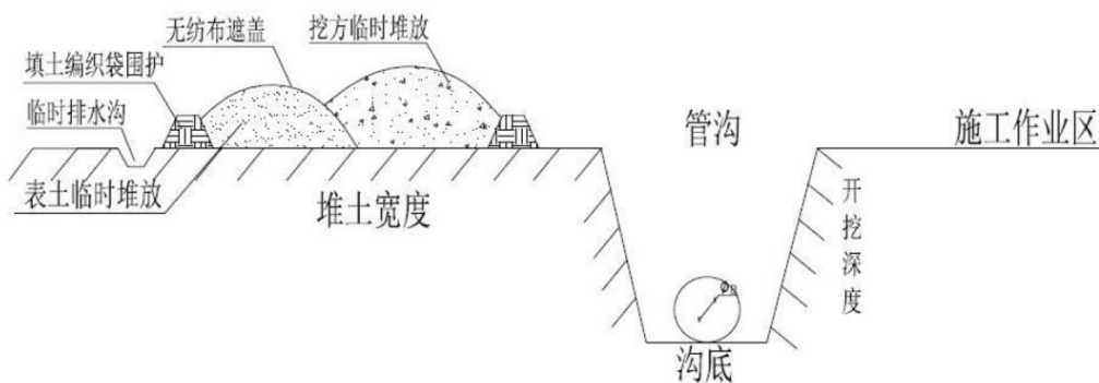
图 2.5-2 管沟及施工作业带典型剖面示意图
