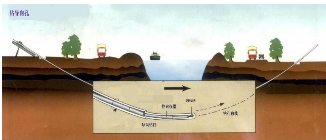
图 2.5-3 钻导向孔示意图
