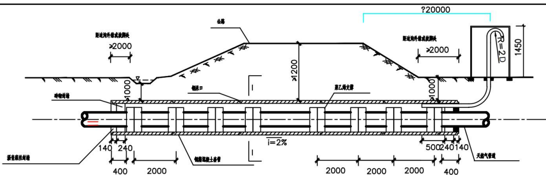
图 2.5-5 一般乡村道路穿越典型纵断面示意图
