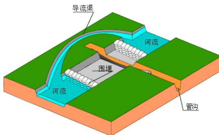
图 2.5-6 水体穿越方案示意图
