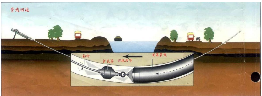
图 2.5-4 拖管示意图
