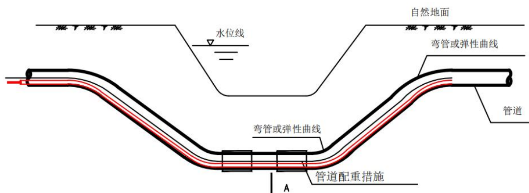
图 2.5-7 水体穿越纵断面示意图
